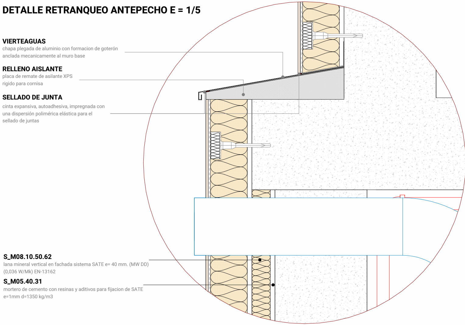
DETALLE RETRANQUEO ANTEPECHO E = 1/5
