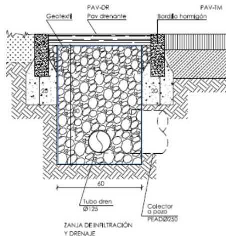
Ejemplo de zanja drenante
