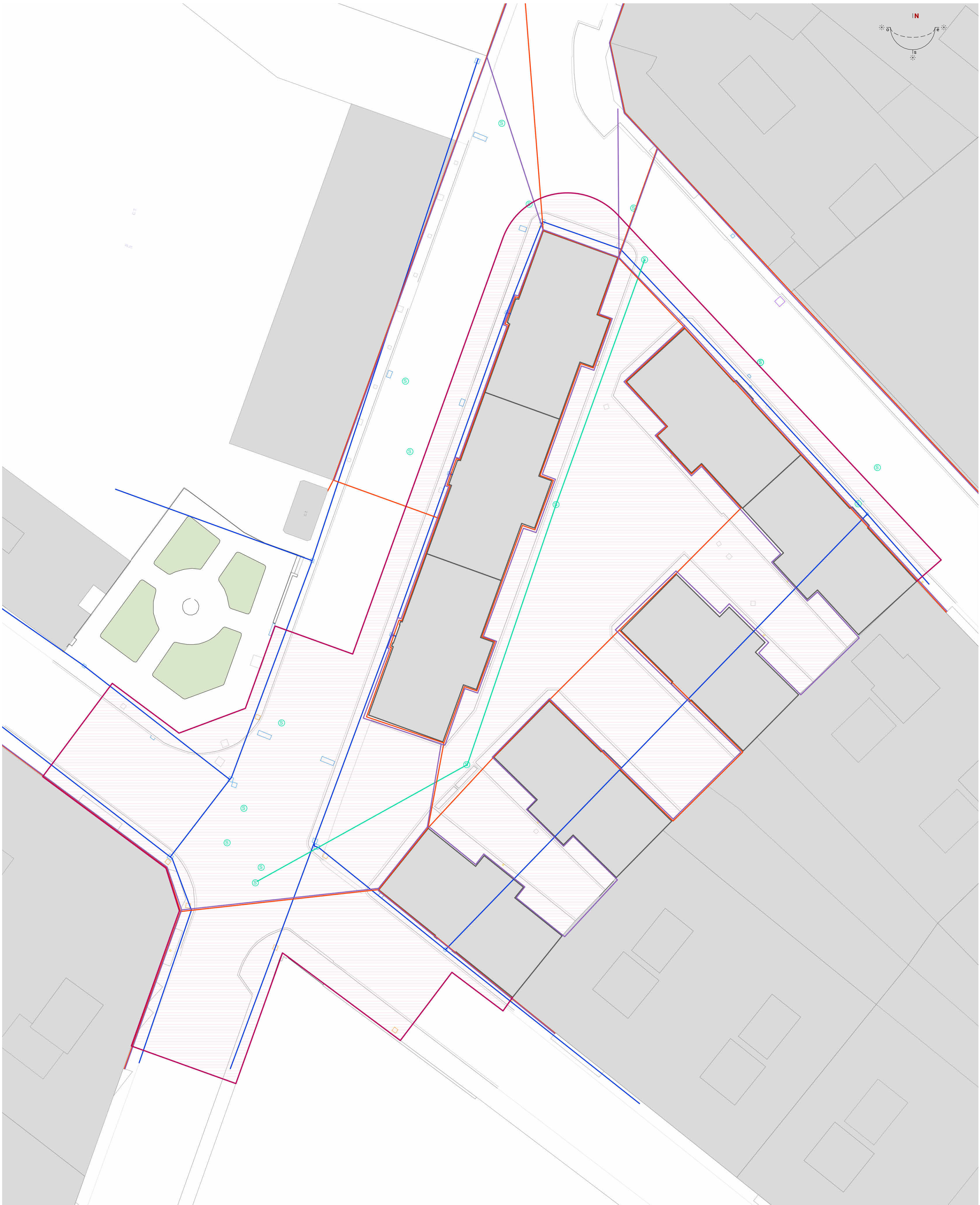
1 U01.01_ESTADO ACTUAL INSTALACIONES U.02.02 e: 1: 200 Coordinación
