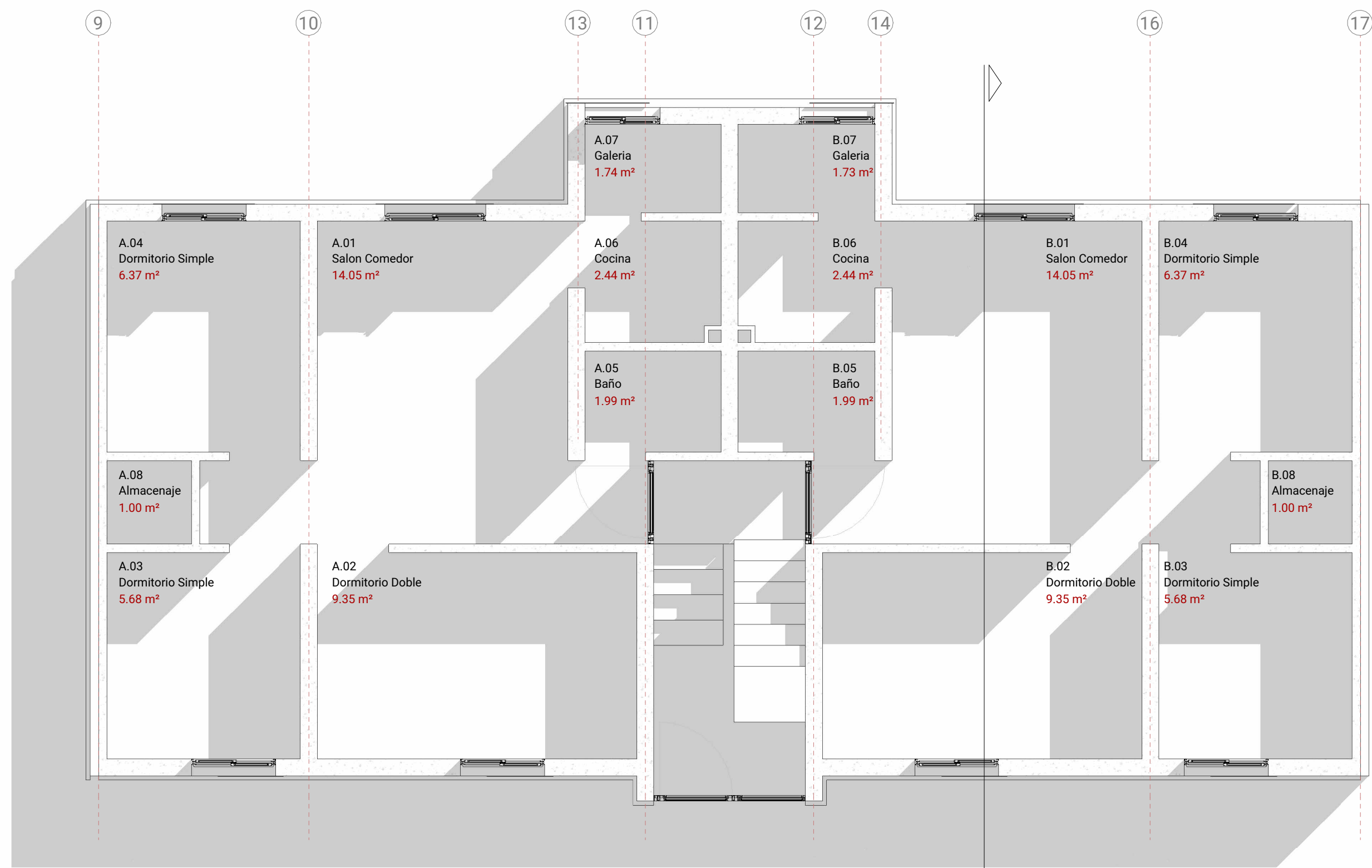
1 S.01.01_PLANTA TIPO ESTADO ACTUAL S.01.01 e/ 1:50 Coordinación
